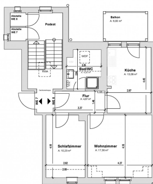
Grundriss DG rechts Wohnung 8 52,7m 2 Wielandstr. 24 04600 Altenburg
